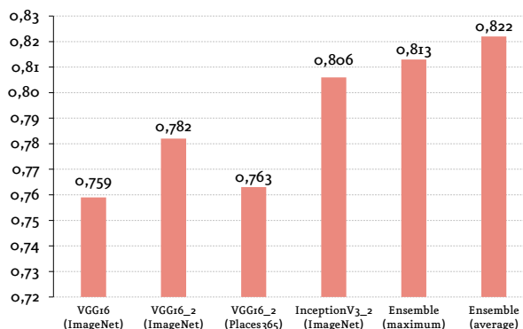
Score F1 para cada arquitectura de red
